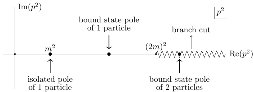
图 50: 全连通传播子的动量表象 \mathfrak{C}(p) 在复 p^2 平面 \mathbb{C}(p^2) 上的解析结构，参考自[19]图 7.3。
