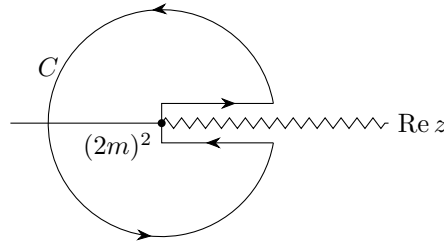
图 51: 复变量 z 绕割线 z \geq 4m^2 的回路 C ，这个回路称为钥匙孔
