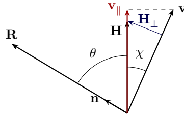
图 49: 速度和磁场的分布图
