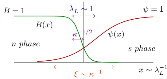
图 38: 无量纲波函数 \psi 和磁场 B 的在 \kappa \ll 1 的渐进分布
