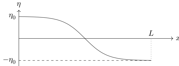
图 21: \eta(x) 的渐进示意图
