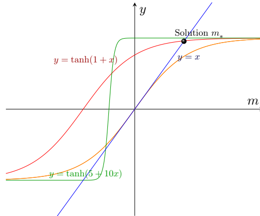
图 7: 自恰性方程的解
