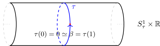
图 44: 一维空间 \mathcal{M}_E = S_\tau^1 \times \mathbb{R} 虚时圆的结构示意图
