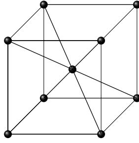
图 5: CsCl分子的晶体结构（体心立方）
