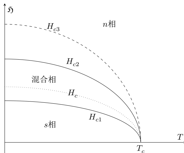
图 39: 二类超导体中各相的临界场的相图
