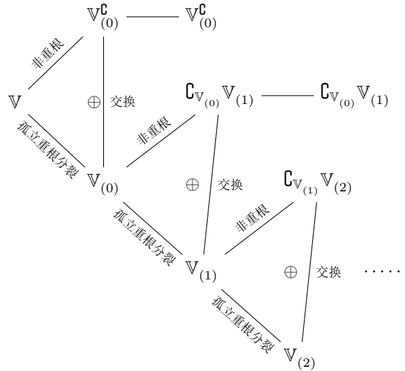
图 47: 微扰导致的向量空间分裂示意图, 此处近似到二阶
