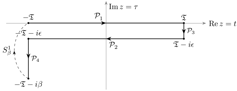
图 45: Konstantinov-Perel路径 z(u) 的构造。
