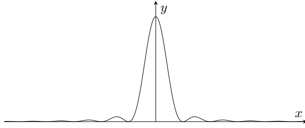
图 48: 函数 \text{sinc}^2(100x) 的图像
