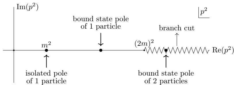
图 51: 全连通传播子的动量表象 \mathfrak{C}(p) 在复 p^2 平面 \mathbb{C}(p^2) 上的解析结构，参考自[19]图 7.3。
