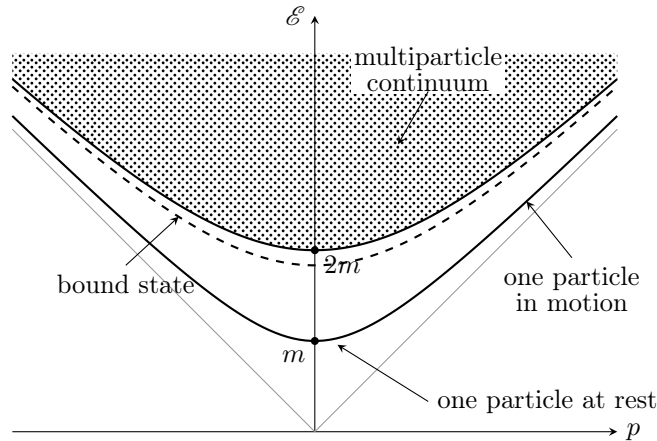
图 50: 时空场典型理论的能谱图，参考自[19]图 7.1。
