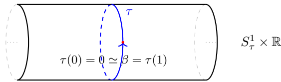
图 44: 一维空间 \mathcal{M}_E = S^1_\tau \times \mathbb{R} 虚时圆的结构示意图
