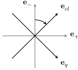
图 46: 坐标系的旋转, 这里令反向支 \mathbf{e}_- 转到对角线。
