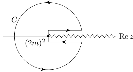
图 52: 复变量 z 绕割线 z \geq 4m^2 的回路 C ，这个回路称为钥匙孔
