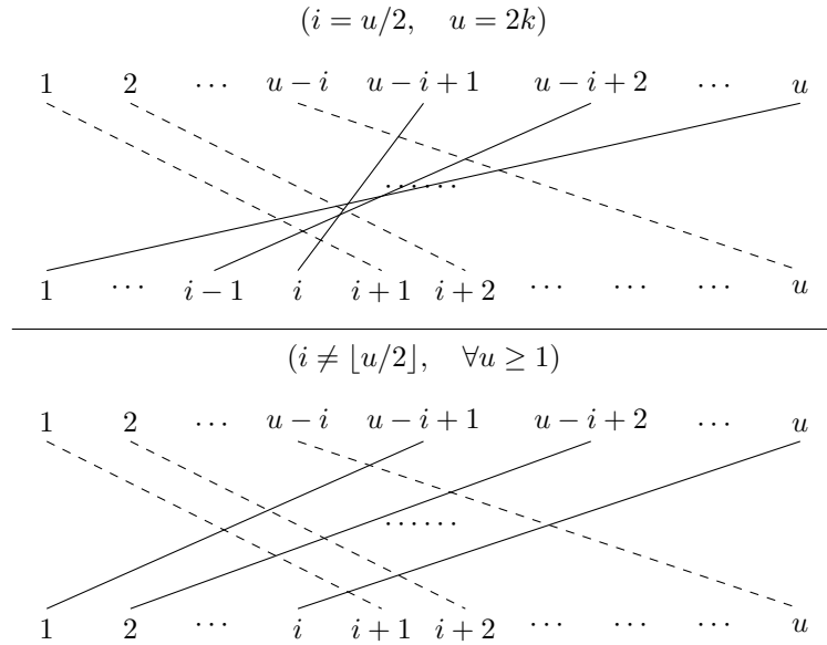
图 49: 缩并规则示意, 图中整数 i \geq 1 对应时空点 x_i , 每一条线对应一个 Feynman 传播子
