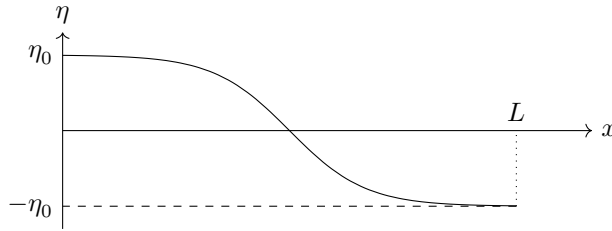
图 21: \eta(x) 的渐近示意图
