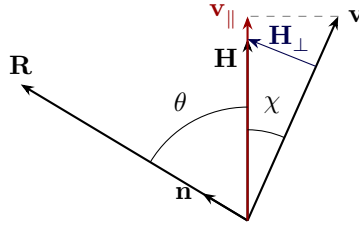
图 50: 速度和磁场的分布图
