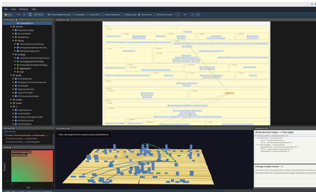
S202: 2D-Abhängigkeitsgraph und 3D-Schichtendarstellung einer Java-Anwendung.
