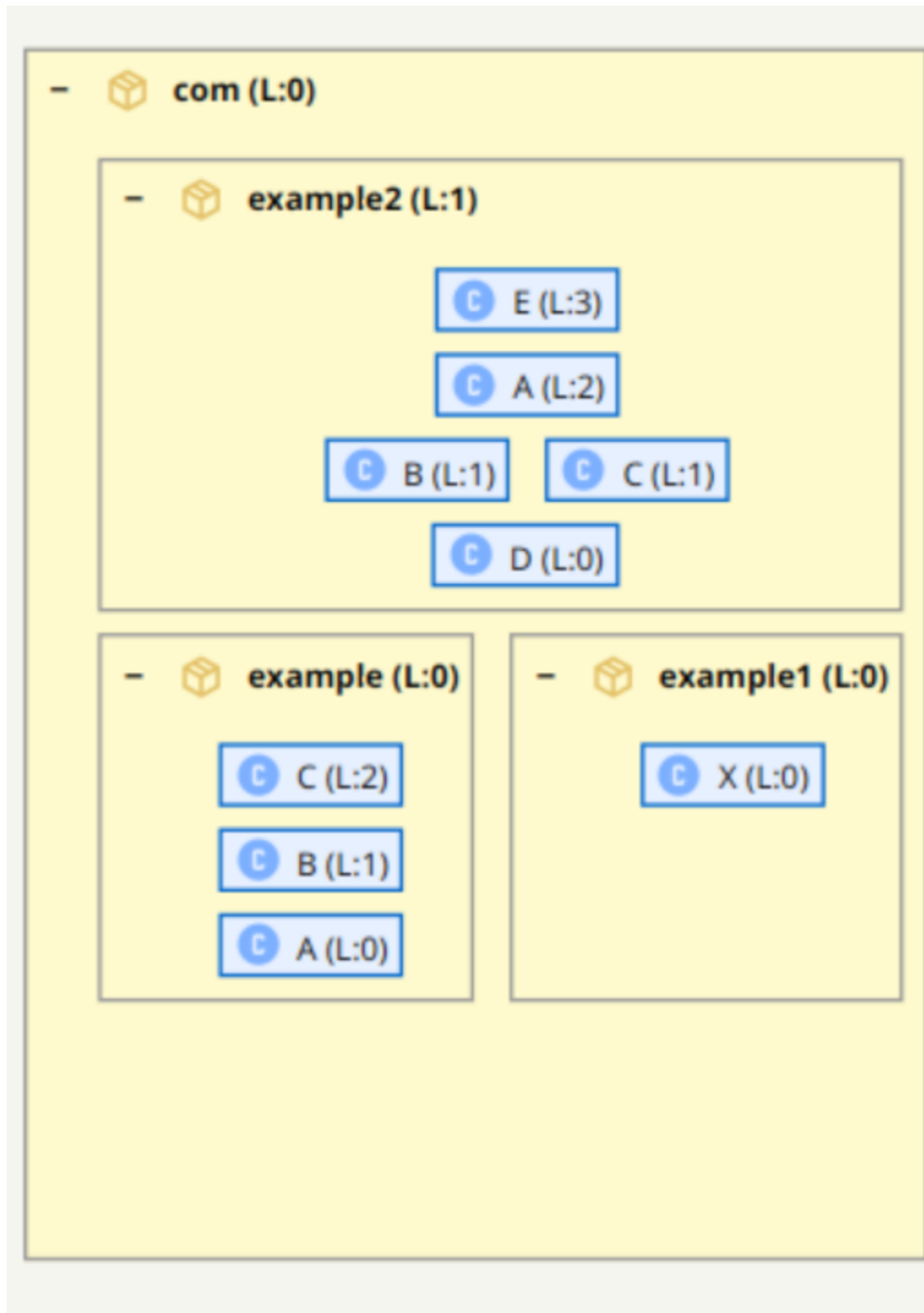
S202-Darstellung mit Paketcontainern und hierarchischer Schichtung.
