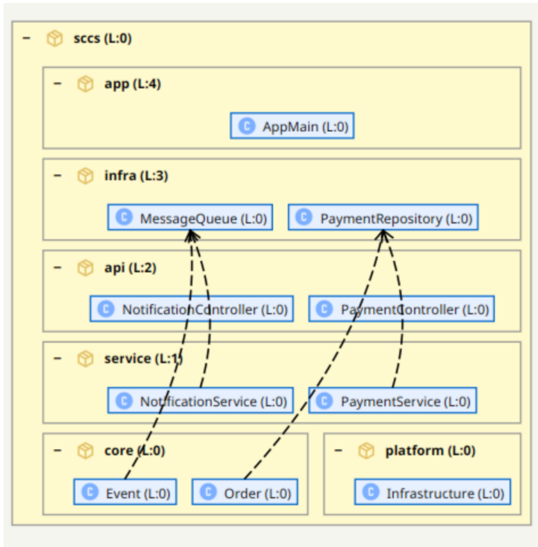
Zyklische S202-Darstellung mit Back-Edges.
