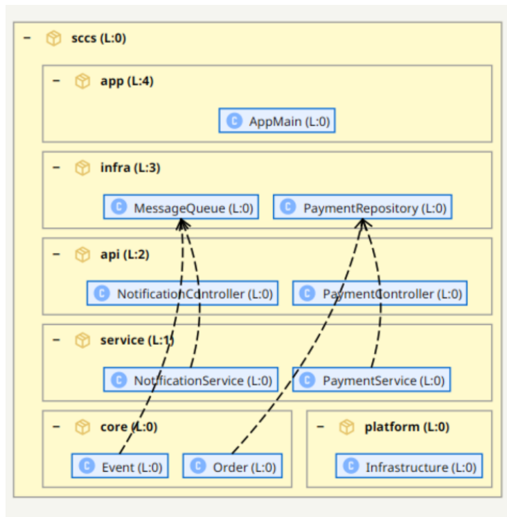
Abbildung 4: Zyklischer S202-Ausschnitt. Die gestrichelten Kanten sind Verletzungen: Sie laufen gegen die aus den Pakatabhängigkeiten abgeleitete Ordnung und bleiben als sichtbarer Befund der Architekturhypothese erhalten. Alle vier gestrichelten Kanten gehören zu den zwei SCCs und werden von S202 als Back-Edges für die Levelberechnung klassifiziert.
