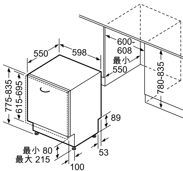
尺寸 (毫米)
