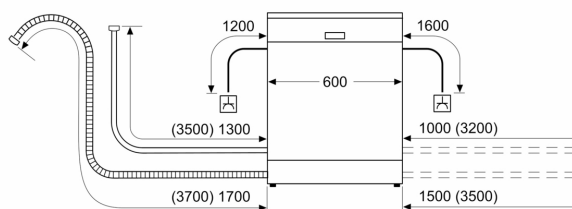
尺寸(毫米)
