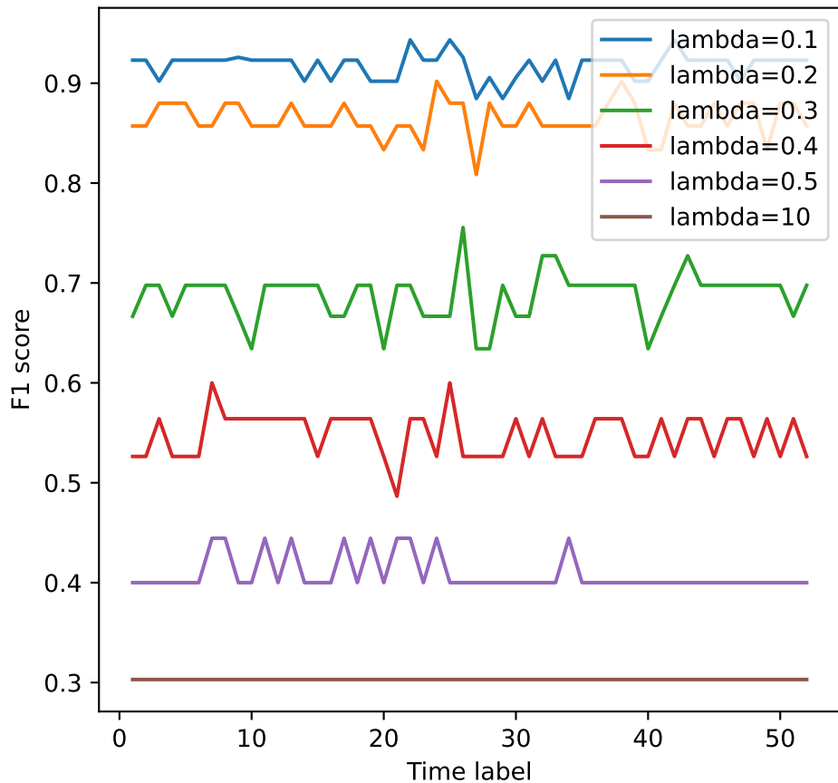
F1 score vs. Time label (msTVGL)
