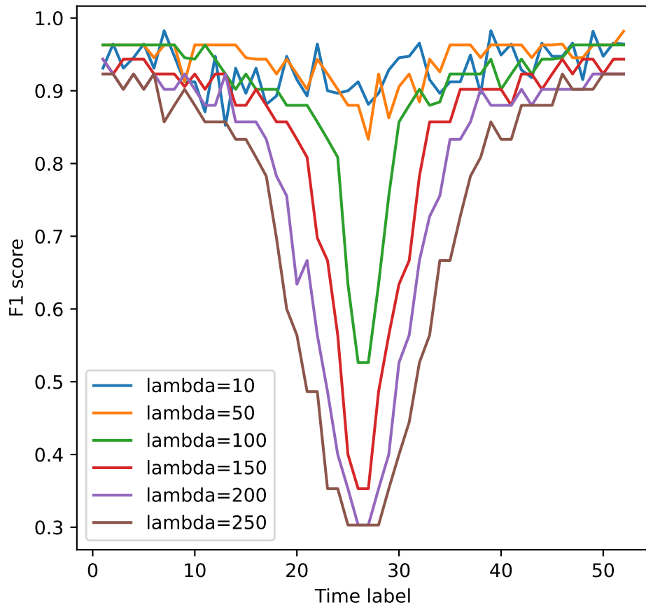
F1 score vs. Time label (TVGL)
