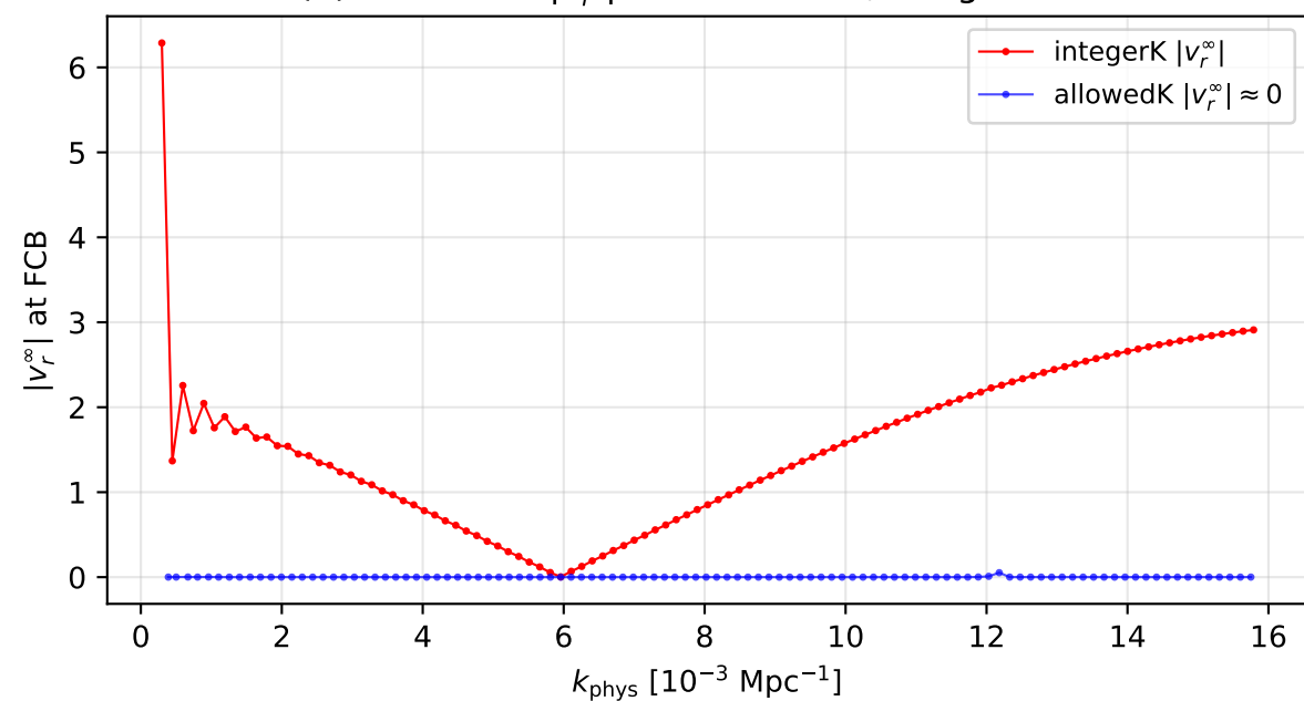
(d) FCB value |v_r^\infty| : allowedK \approx 0 , integerK \neq 0
