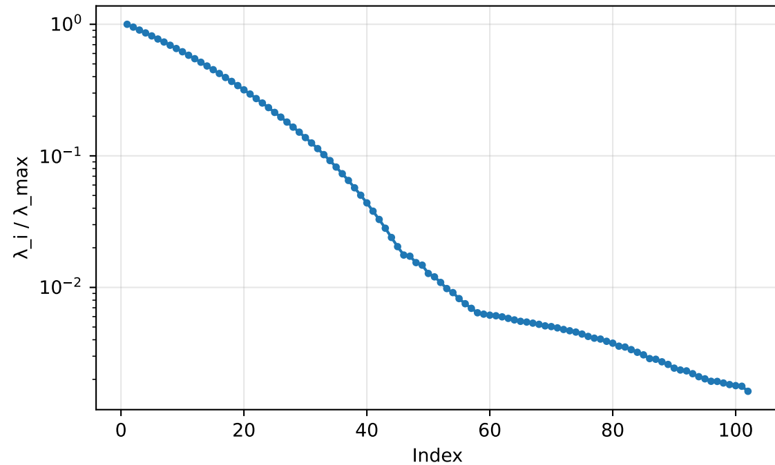
Gram eigenvalue spectrum: G1 (integerK)
