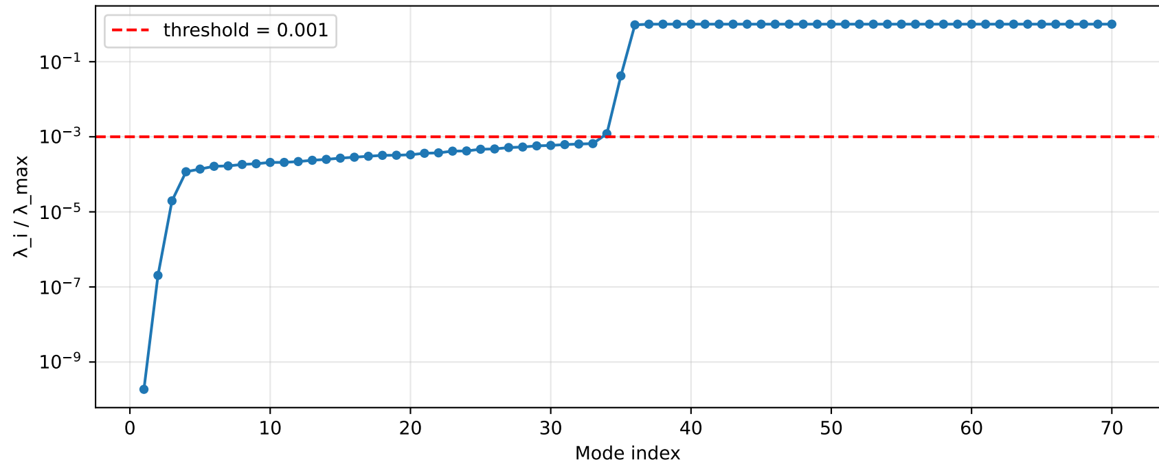
Matching-solution eigenvalue spectrum
