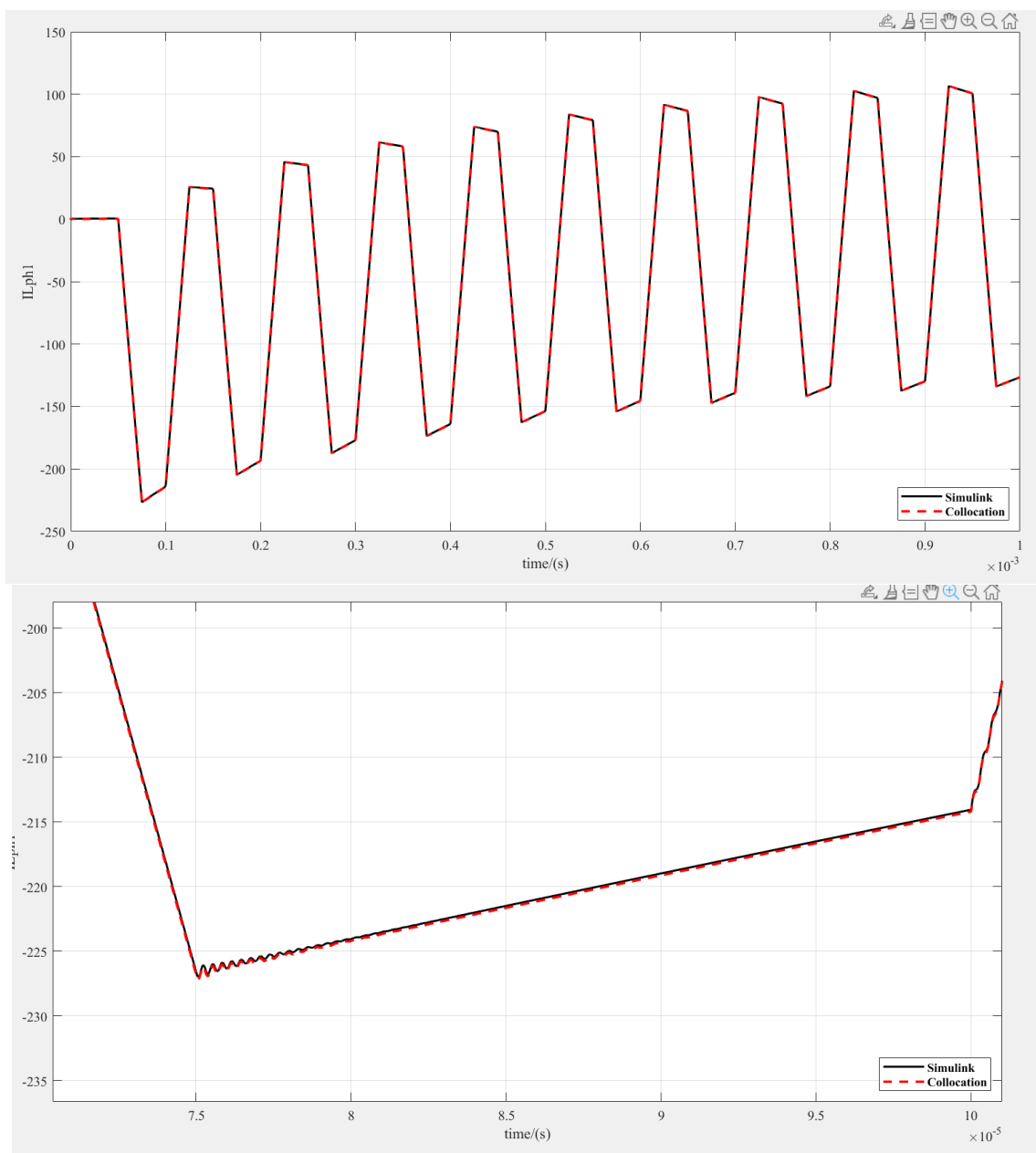
图 5: IL_{ph1} -时间图像
