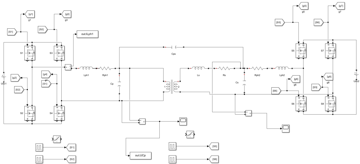
图 1: simmulink模型
