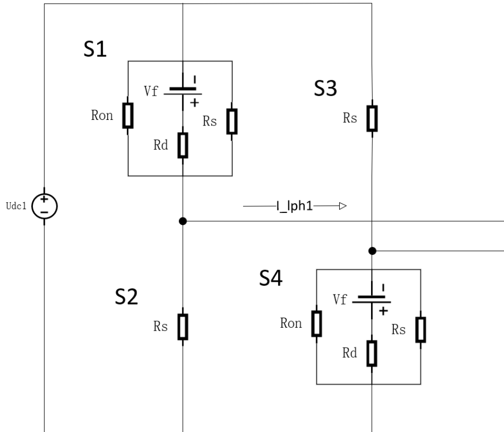
图 3: 控制信号(g1,g2,g3,g4)=(1,0,0,1)情况
