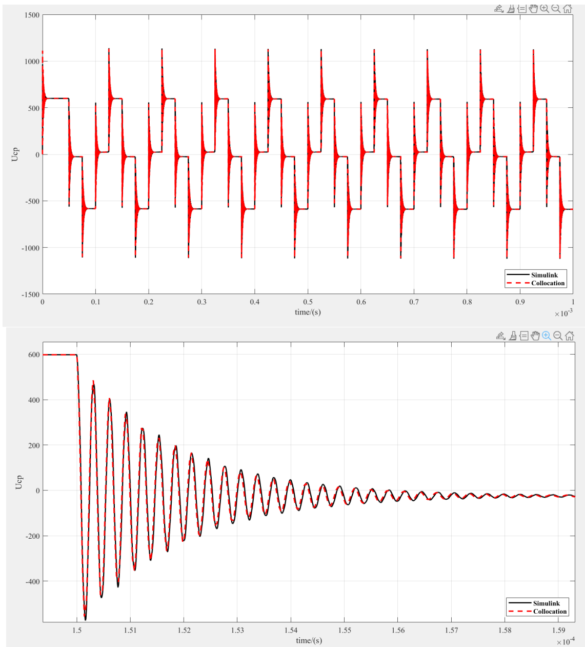
图 4: U_{cp} -时间图像
