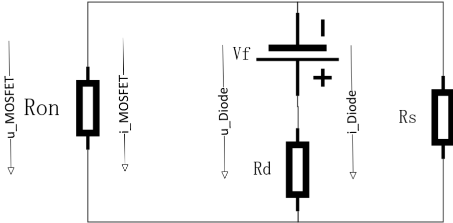
图 2: MOSFET和Diode示意图
