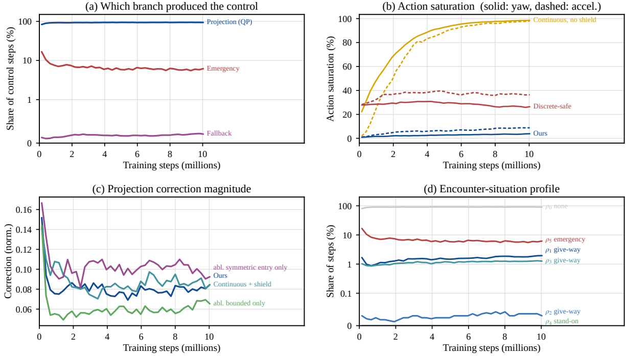
Figure 5 安全盾的行为随训练演化，取自训练期遥测。（a）本文方法中每一步控制由哪一支产生（对数纵轴）。（b）动作饱和率，转艏轴与加速度轴分开，有界分布、无界高斯与离散网格叠于同图；离散网格的动作上界恰等于连续动作箱半宽，故两者共用同一条打满判据。（c）投影修正量，按动作箱半宽归一化。（d）会遇态势占比（对数纵轴）；直航态 \rho_4 在本场景库上几乎不触发，逐段中位数为零，故其曲线贴在零线上。本图为训练期采集，与表 6 的评估口径不同。
