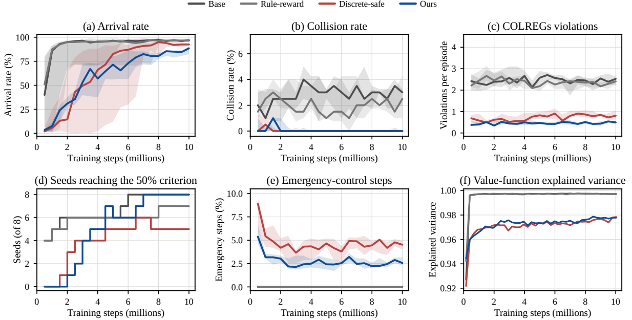
Figure 4 样本效率与训练可靠性，横轴为训练步数，四种主对照配置共用图例；粗线为跨种子中位数，阴影为四分位距。横轴自第一个评估点（0.5 百万步）起画——训练期没有零步评估，补一个原点会是凭空添加的数据点。（a）到达率。（b）碰撞率。（c）每局 COLREGs 违规。（d）到达率达到收敛判据的种子数。（e）紧急控制步占比。（f）值函数可解释方差。消融配置不入本图，其对照见图 3。离散安全基线尚有两颗种子在训练（分别跑到第 14、13 段），其中位线在末段由较少种子构成，逐种子细线的长度即为各自的实际进度。纵轴为 100 个验证场景上的数值，与表 4 的官方测试集口径不同。
