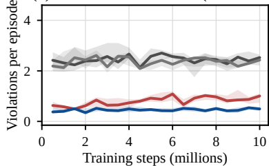
(d) COLREGs violations (validation)
