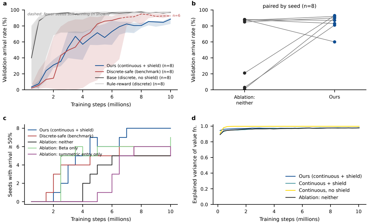
Figure 4 样本效率与训练可靠性样本效率与训练可靠性，横轴为训练步数。（a）四种主对照配置的验证集到达率，实线为跨种子中位数、阴影为四分位距；虚线段表示该配置尚有种子在训练，参与统计的种子数已在线端标出。（b）同种子配对，消融·两项都不改→本文方法。（c）到达率达到收敛判据的种子数。（d）值函数可解释方差。纵轴为100个验证场景上的数值，与表6的官方测试集口径不同。
