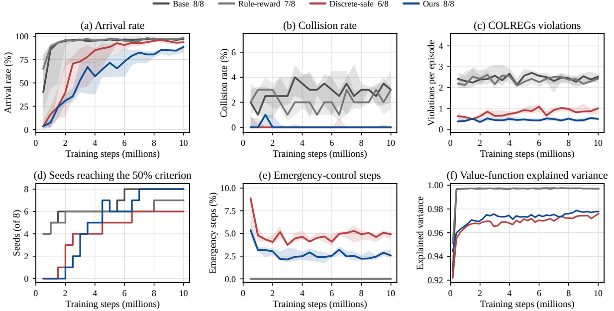
Figure 4 样本效率与训练可靠性，横轴为训练步数，四种主对照配置共用图例，图例中的 n/8 为该配置的收敛种子数。粗线为中位数、阴影为四分位距，二者均只统计收敛种子——发散种子会把分位带拉到零，而“有多少种子练得成”这件事由 (d) 单独回答。(d) 计入全部 8 颗种子。横轴自第一个评估点（0.5 百万步）起画，训练期没有零步评估，补一个原点会是凭空添加的数据点。(a) 到达率。(b) 碰撞率。(c) 每局 COLREGs 违规。(d) 到达率达到收敛判据的种子数。(e) 紧急控制步占比。(f) 值函数可解释方差。消融配置不入本图，其对照见图 3。离散安全基线有一颗种子在第 19 段后中断，其余 71 条 run 均跑满 20 段；逐种子细线的长度即为各自的实际进度。纵轴为 100 个验证场景上的数值，与表 4 的官方测试集口径不同。
