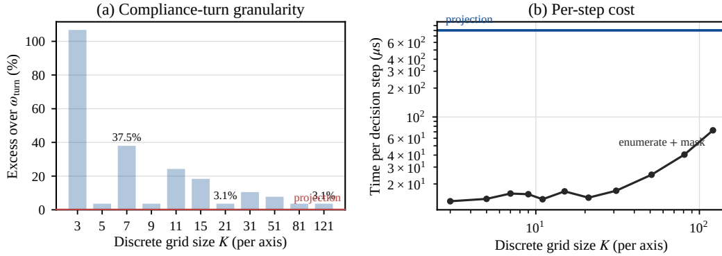
Figure 7 投影替代枚举的收益与代价。（a） K \times K 网格能取到的最小合规转艏率比下确界 \omega_{turn} 高出的比例，由网格步长与 \omega_{turn} 的整除关系决定，不随 K 单调下降；连续动作加投影恰好取到下确界（红线）。（b）单个决策步的耗时，枚举屏蔽随 K^2 增长，投影与 K 无关。（a）为精确算术，（b）为单机实测，只用于比较随 K 的增长关系，不是论文报数用的部署耗时。
