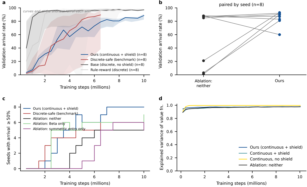
Figure 4 样本效率与训练可靠性。全部取自训练期记录，横轴为训练步数。（a）四种主对照配置在 100 个验证场景上的到达率学习曲线（每 507,904 步一个点），实线为跨种子中位数、阴影为四分位距；各条曲线止于该配置最短的那个 run。（b）同种子配对：消融·两项都不改 \rightarrow 本文方法，每条折线一颗种子。（c）到达率达到收敛判据（第 5.2.3 节）的种子数随训练步数的变化。（d）值函数可解释方差，用于区分“还在爬”与“已经崩”。曲线未做平滑，仅按训练步数分箱取中位数。注意：本图的到达率为 100 个验证场景上的数值，与表 5 的官方测试集口径不同，不可互相引用。
