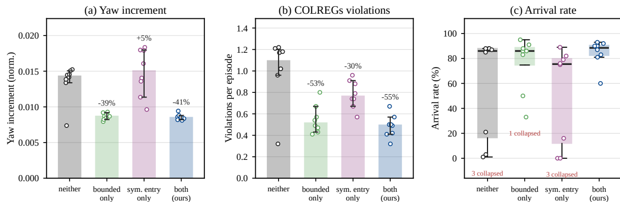
Figure 3 两项改进的贡献拆解（ 2 \times 2 消融，同种子配对）。（a）（b）柱为跨种子中位数，误差棒为按种子重采样的自助法 95% 区间，柱顶给出相对最左一柱的变化、配对 Wilcoxon 符号秩检验的显著性记号与同向种子数。（c）到达率的分布是双峰的（部分种子发散），故改用箱线图，发散种子数标于箱下。每格的空心点均为单颗种子。本图为验证集 100 场景上的数值，与表 4 的官方测试集口径不同；违规为直航与让路之和。
