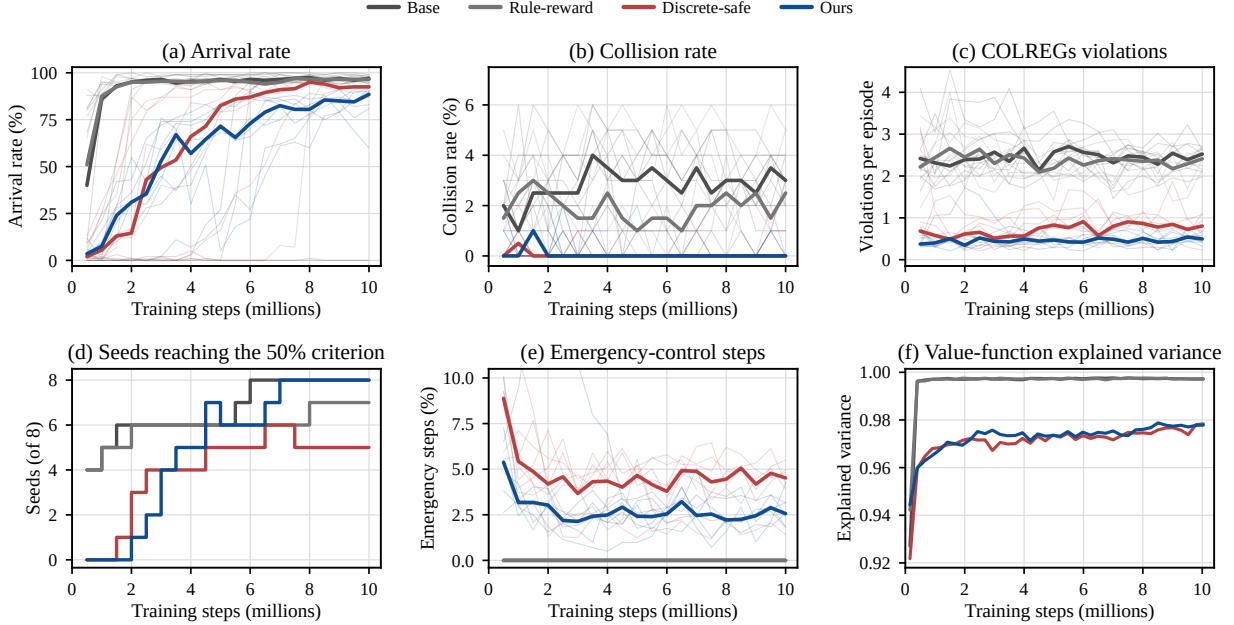
Figure 4 样本效率与训练可靠性，横轴为训练步数，四种主对照配置共用图例；细线为单颗种子、粗线为跨种子中位数。（a）到达率。（b）碰撞率。（c）每局 COLREGs 违规。（d）到达率达到收敛判据的种子数。（e）紧急控制步占比。（f）值函数可解释方差。消融配置不入本图，其对照见图 3。离散安全基线尚有两颗种子在训练（分别跑到第 14、13 段），其中位线在末段由较少种子构成，逐种子细线的长度即为各自的实际进度。纵轴为 100 个验证场景上的数值，与表 4 的官方测试集口径不同。
