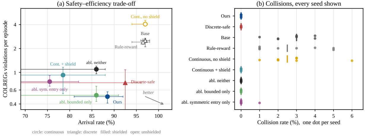
Figure 2 安全—效率权衡。 （a）横轴为到达率、纵轴为每局 COLREGs 违规数（对数轴），点为跨种子中位数，误差棒为按种子重采样的自助法 95% 区间，右下角为理想区；圆为连续动作、三角为离散动作，实心为带盾、空心为无盾。（b）碰撞率逐种子画出，一点一颗种子，短竖线为中位数。误差棒之所以宽，是因为每条臂都含发散种子，见第 5.2.3 节的“仅收敛种子”一版。本图为验证集 100 场景上的数值，与表 6 的官方测试集口径不同；违规为直航与让路之和，拆分值训练期不回传。三条外部几何基线不训练、无训练期产物，故不在本图内。
