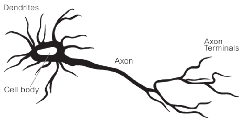
Figura 3.1: Modelo do neurônio biológico. Fonte [32].
