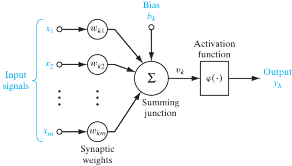
Figura 3.2: Modelo do neurônio artificial. Fonte [33].
