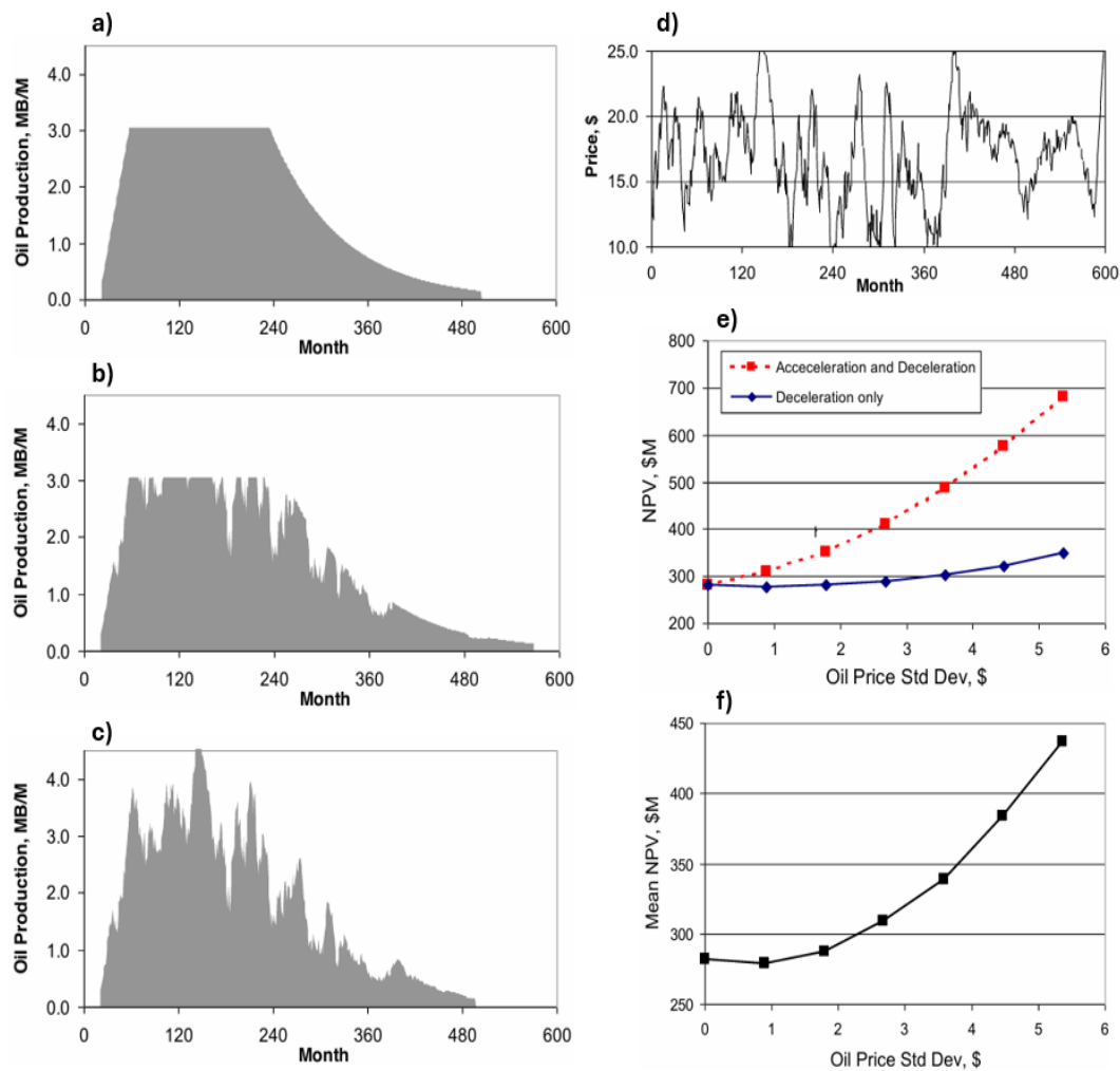
Figura 2.14: Valor da flexibilidade. Fonte [11].
