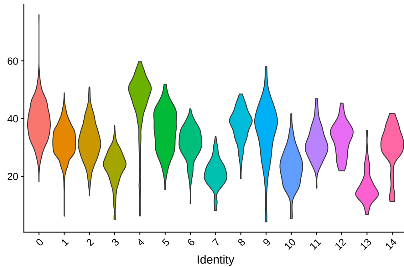
Ribosomal %
