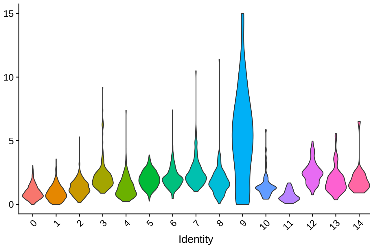
Mitochondrial %
