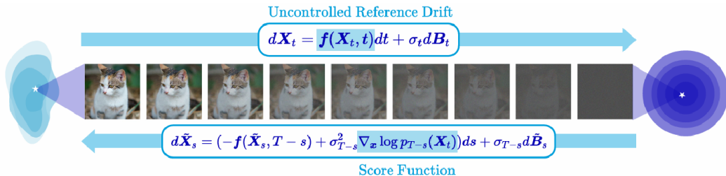
圖: Score-based 擴散模型。注意：下方公式的 \mathbf{X}_t 應理解為 \tilde{\mathbf{X}}_s 。圖源：Figure 7 [T26]。
