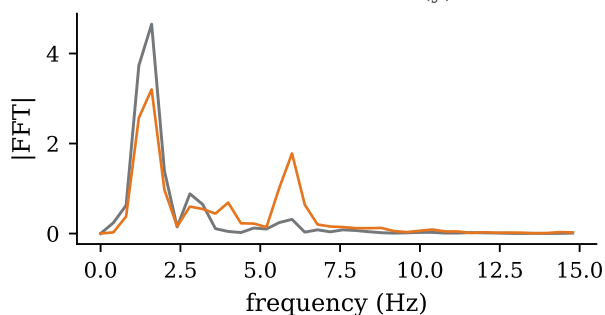
Marker 13 — FFT(y)
