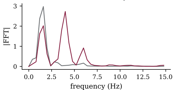
Marker 9 — FFT(y)
