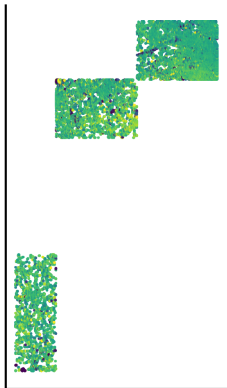
LASSO error
