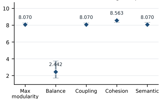
(b) Cohesion
