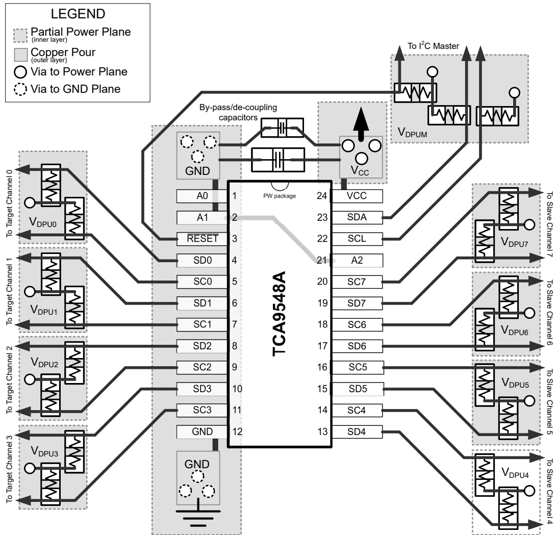
图 8-8. Layout Schematic
