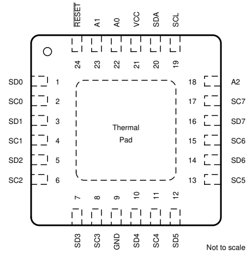
图 4-2. RGE Package, 24-Pin VQFN (Top View)
