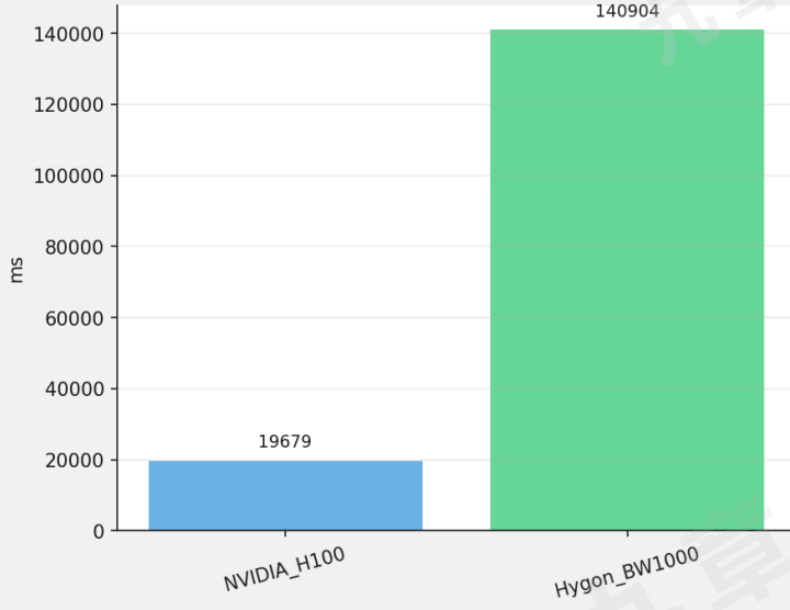
TTFT P99 (ms)
