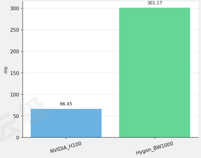
TPOT P99 (ms)
