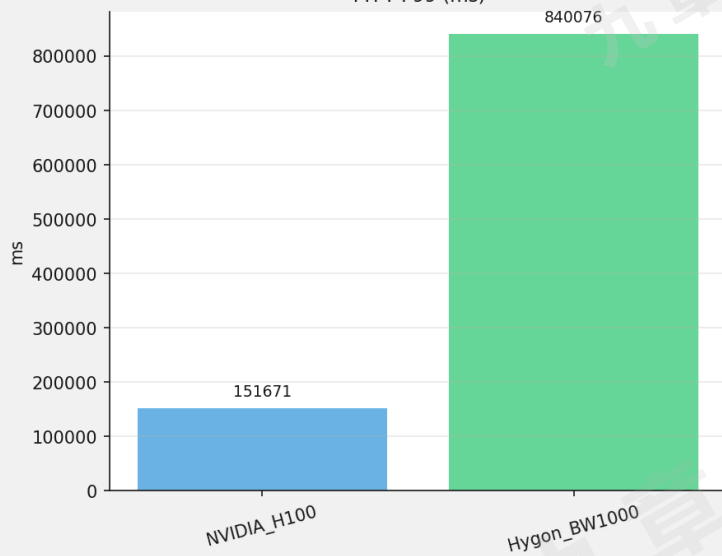
TTFT P99 (ms)
