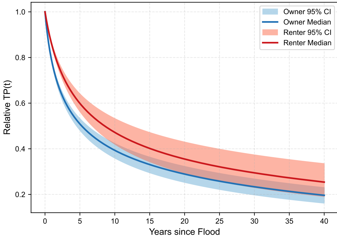
Bootstrap Parameter Uncertainty (N=100)
