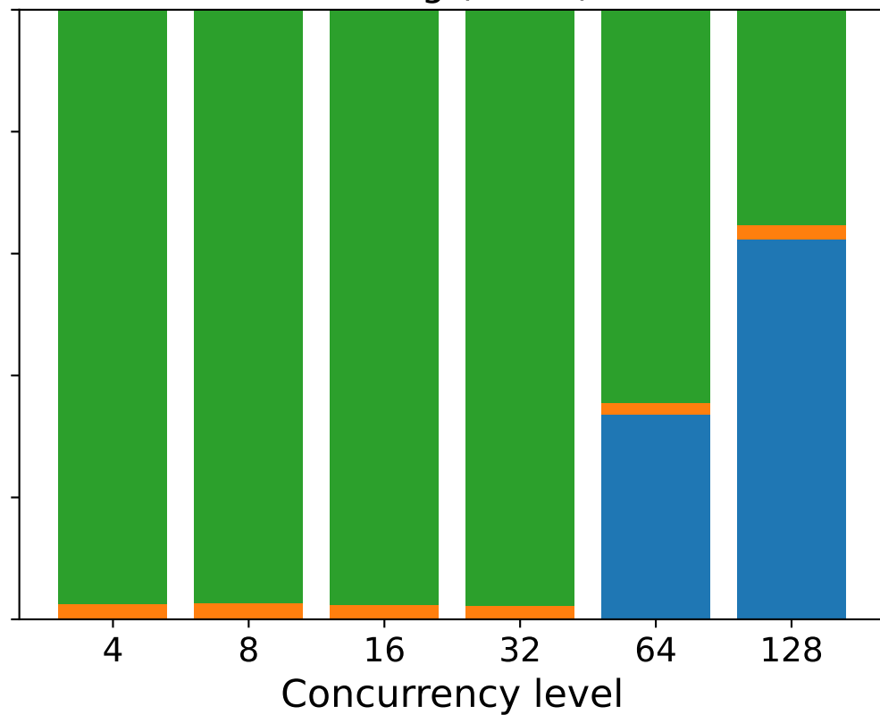
Coding (MBPP)
