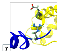
ARG134-GLU92
