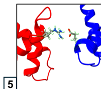
GLU142-ARG79
