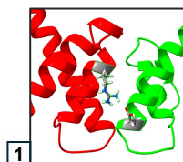
GLU74-ARG96
