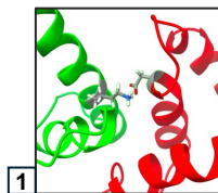
LYS49-ASP71
