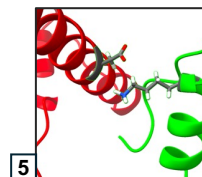
LYS91-ASP65
