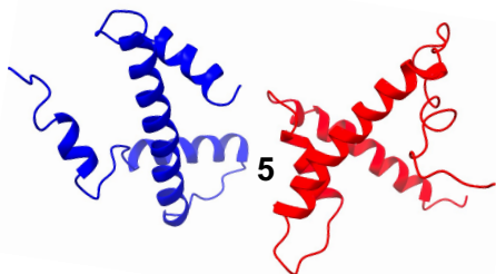
GLU142-ARG79
