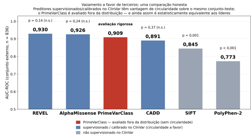
Figura 6. Comparação honesta com o estado da arte: preditores supervisionados/calibrados em ClinVar (azul) têm circularidade a favor; o modelo-carro-chefe (vermelho) é avaliado fora da distribuição.
