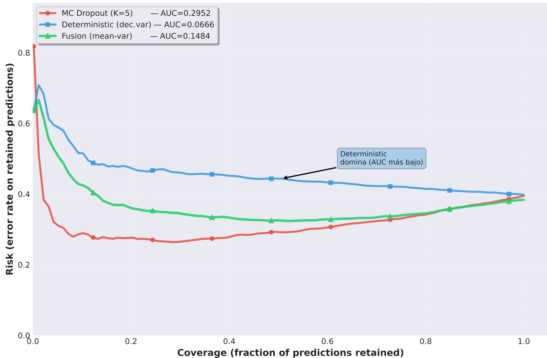
Figure RQ7.1: Risk-Coverage Curves (datos reales — nivel detección)
