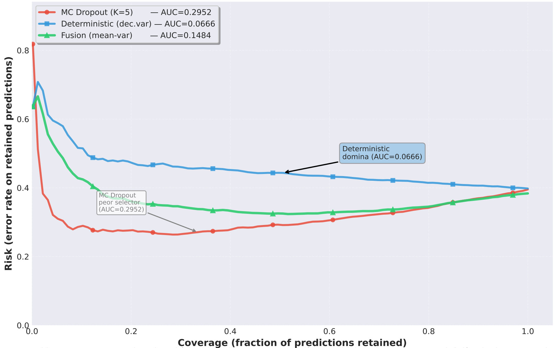
Figure RQ7.1: Risk-Coverage Curves (datos reales — nivel detección) Deterministic domina (AUC más bajo = mejor selector de incertidumbre)
