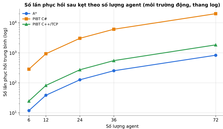
Hình 4.27: Số lần phục hồi sau kết theo số lượng agent (môi trường động, thang logarit)
