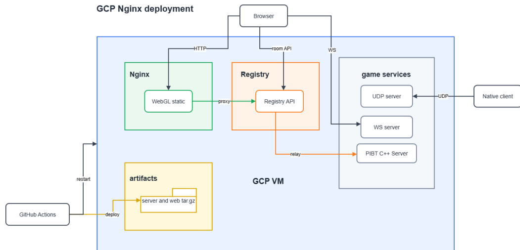
Hình 4.21: Sơ đồ triển khai WebGL qua GCP/Nginx và các dịch vụ trò chơi
