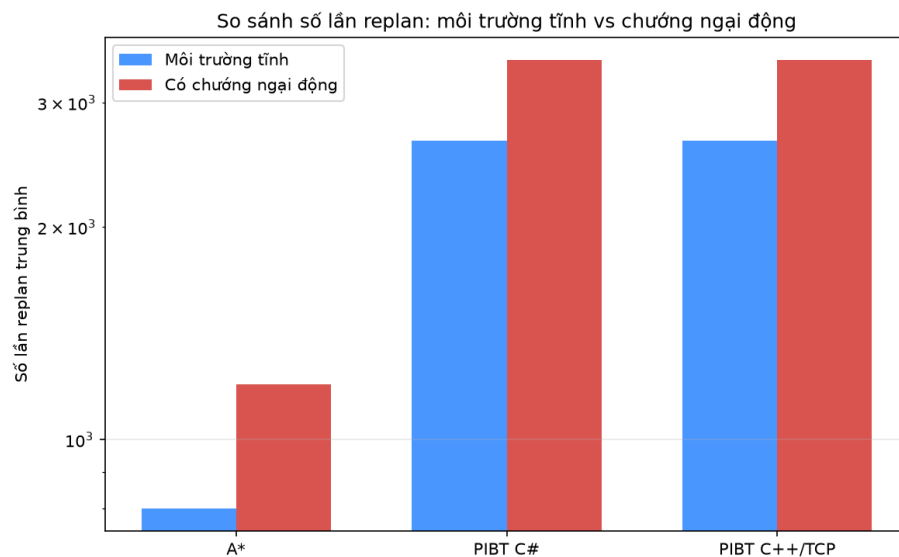
Hình 4.20: So sánh số lần tái hoạch định giữa môi trường tĩnh và có chương ngại động
