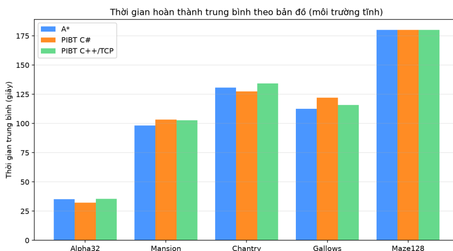
Hình 4.18: Thời gian hoàn thành trung bình theo bản đồ (môi trường tĩnh)
