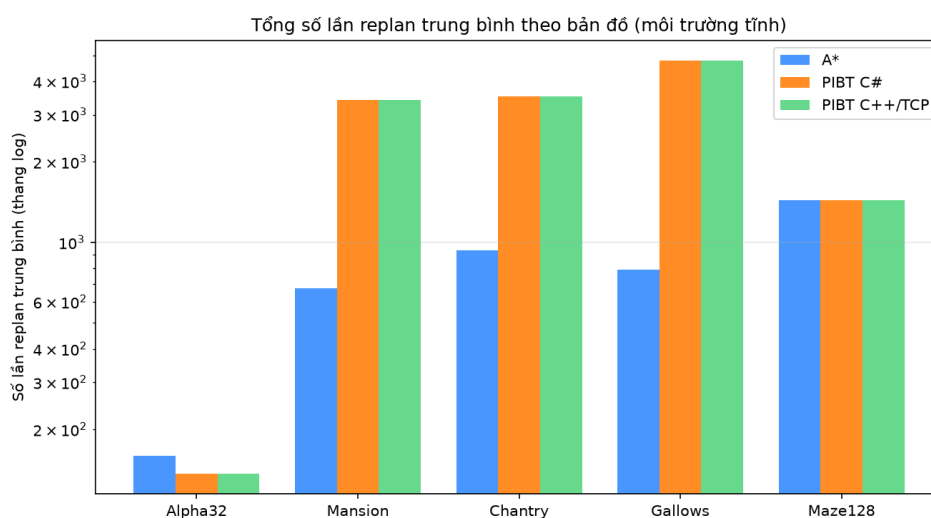
Hình 4.19: Tổng số lần tái hoạch định trung bình theo bản đồ, thang logarit (môi trường tĩnh)
