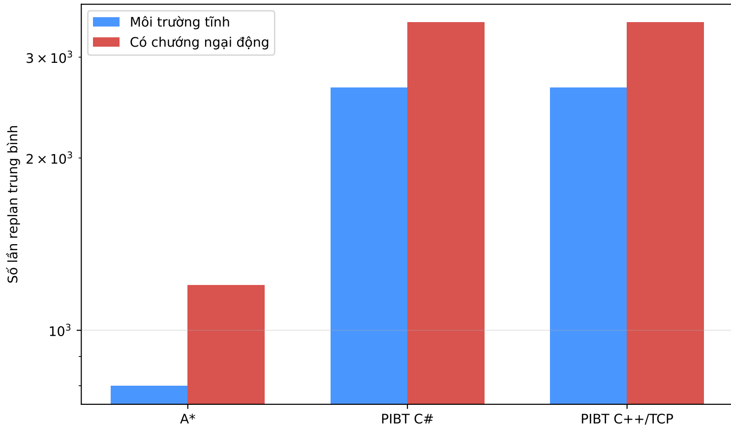
So sánh số lần replan: môi trường tĩnh vs chương ngại động
