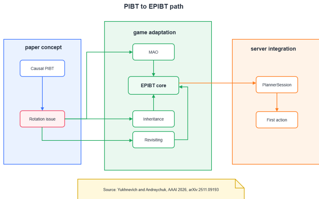
Hình 5.4: Lộ trình chuyển từ PIBT sang EPIBT cho Enemy Agent: khái niệm trong bài báo (vấn đề xoay hướng), phân tích ứng cho game (multi-action operation, kế thừa operation) và phân tích hợp máy chủ (phiên lập kế hoạch, trả về hành động đầu tiên)
