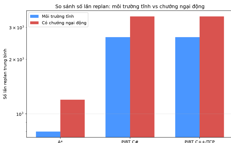
Hình 4.20: So sánh số lần tái hoạch định giữa môi trường tĩnh và có chương ngại động
