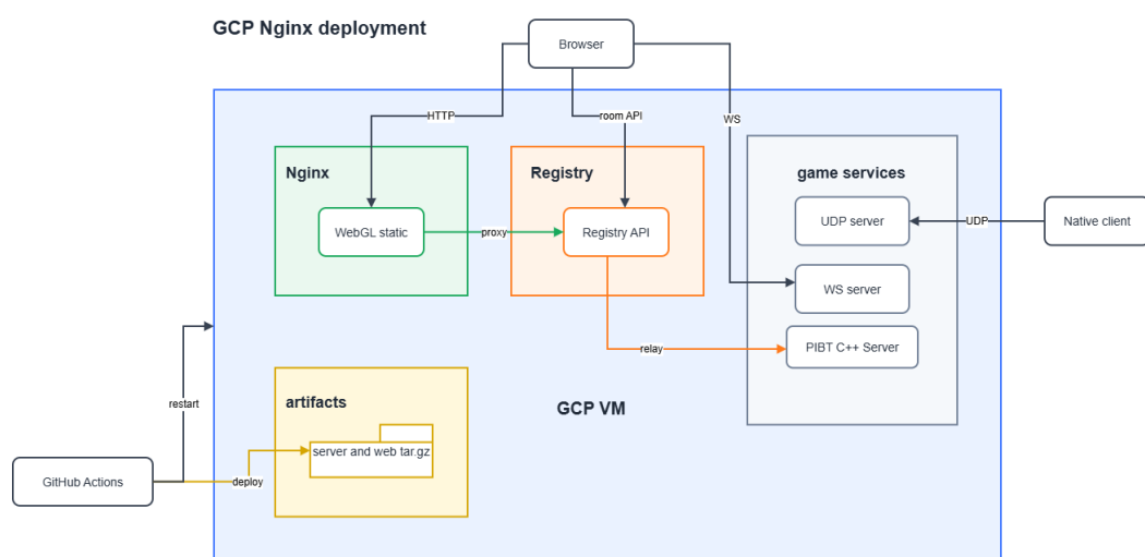
Hình 4.21: Sơ đồ triển khai WebGL qua GCP/Nginx và các dịch vụ trò chơi
