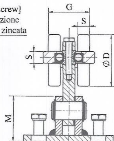
SEZIONE A-A [SECTION A-A]
