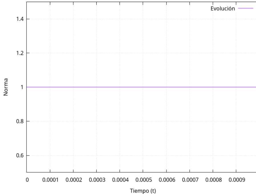
Figura 2: Evolución de la norma de la función de onda a lo largo del tiempo.
