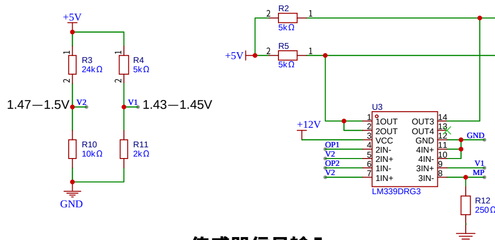
传感器信号输入
