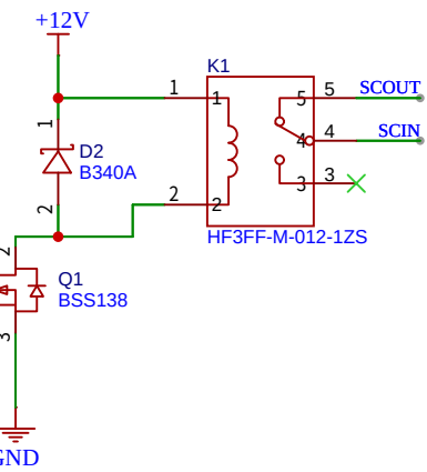
安全回路进入和输出
