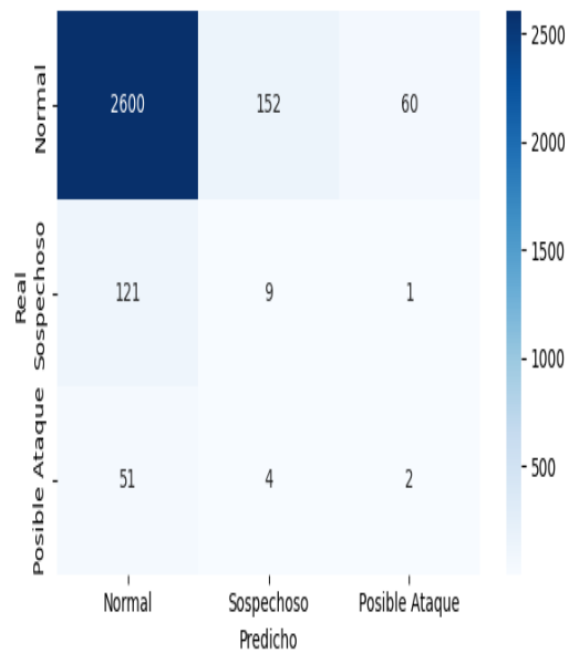
Matriz de Confusión - RF
