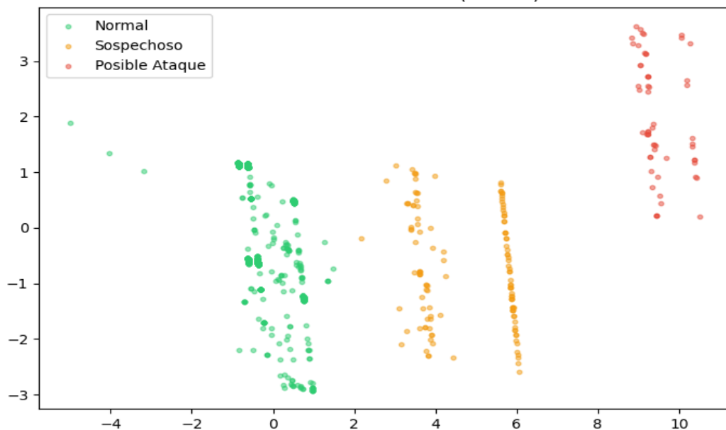
Visualización de Clusters (PCA 2D)
