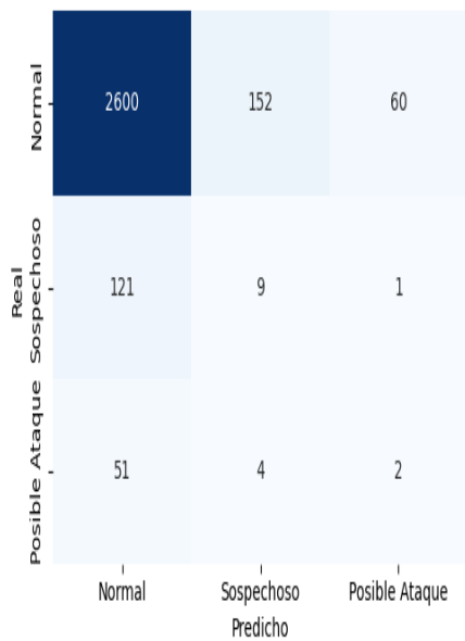
Matriz de Confusión - MLP
