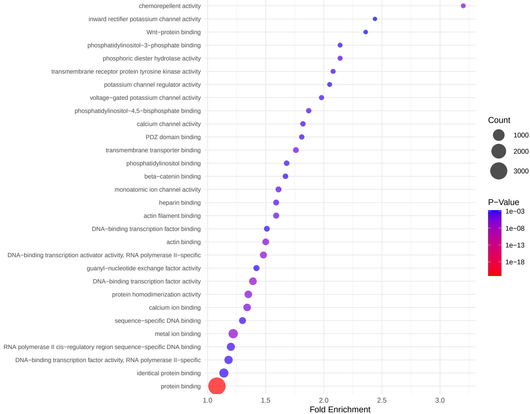
PRAD_WhiteRace_DownRegulated_MFDirect_Dotplot
