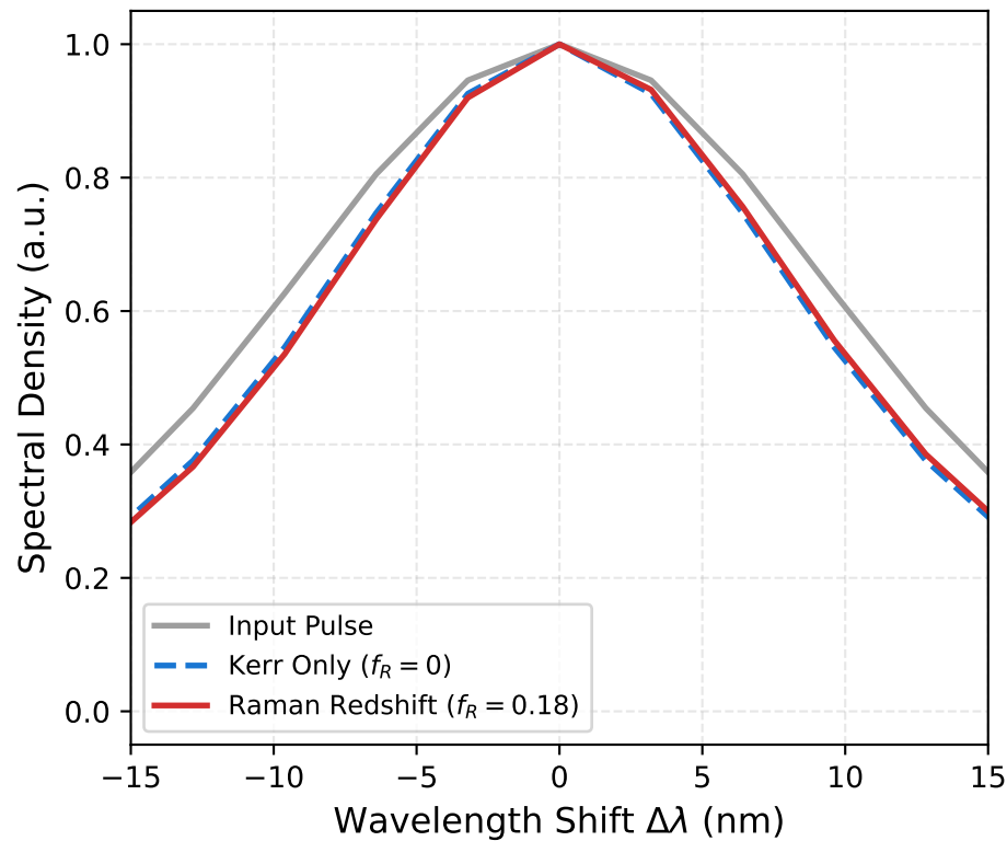
(b) Raman Redshift ( z = 40 m)
