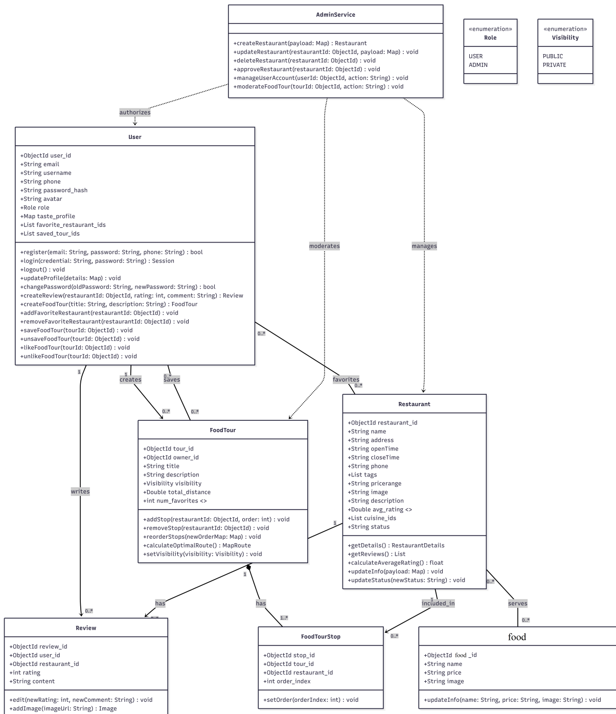
Hình 4.16: Class Diagram
